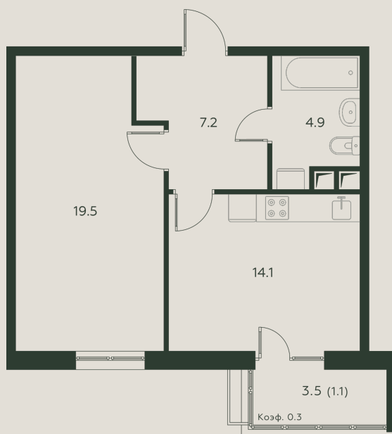
Размеры
